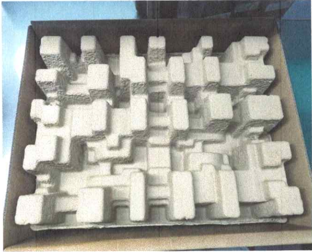
2.在下层鸡蛋壳放满 3pcs 的 PA04394 后，如图所示盖上层鸡蛋壳和外箱盖子
